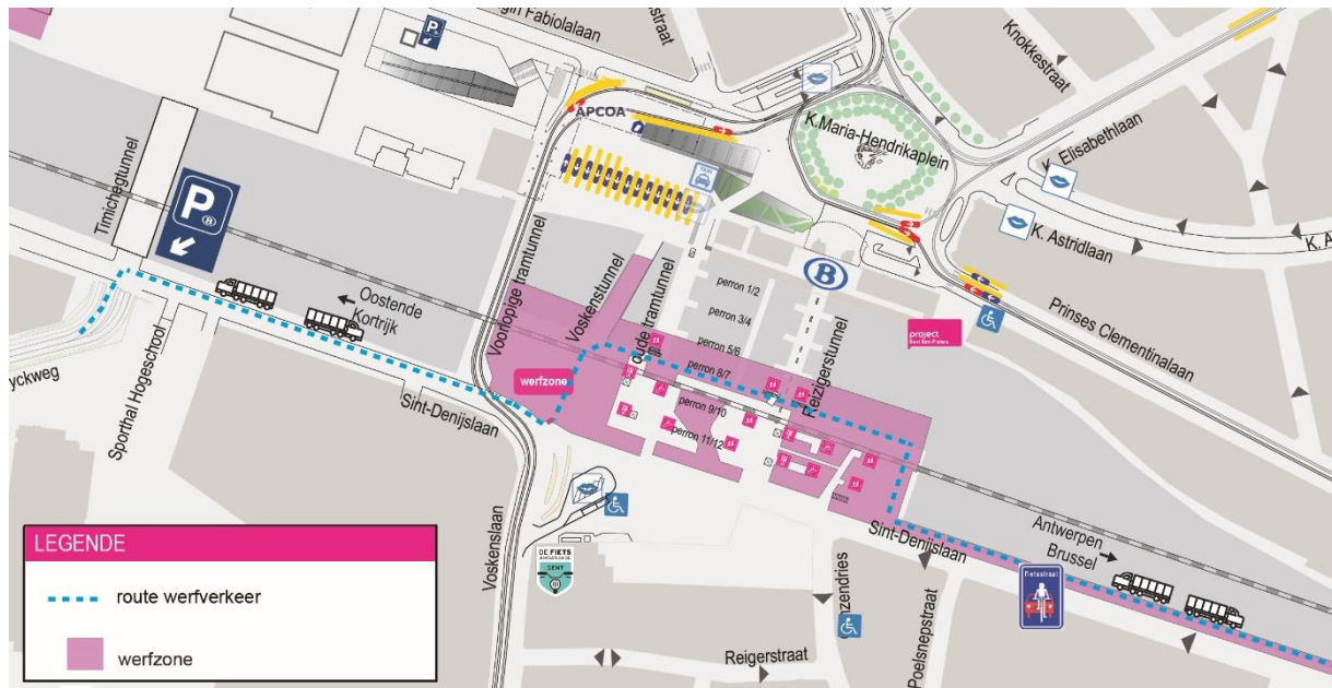
Overzichtsaanpak met de werfzone en de routes van het werfverkeer
