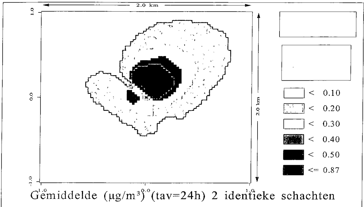
Figuur 3: grafiek van de jaargemiddelde PM 10 concentraties door toedoen van de parking (piek scenario, wagenpark 2003, resolutie 25 m, gemiddelde meteo).
