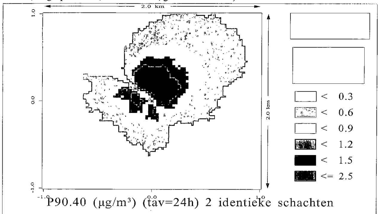
Figuur 4: grafiek van de 90,4 de percentiel van de daggemiddelde PM 10 concentraties door toedoen van de parking (piek scenario, wagenpark 2003, resolutie 25 m, gemiddelde meteo).
